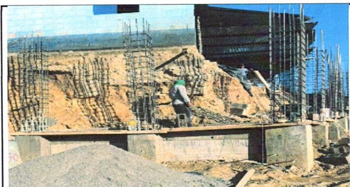
Foto 5: se observa la fundición de la primera solera y columnas del Mejoramiento de muro de contención con concreto lanzado y drenes
