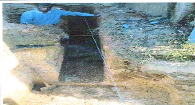
Foto1: Se aprecia el inicio de sanjeo para el cimiento del muro de contención con concreto lanzado y drenes.
